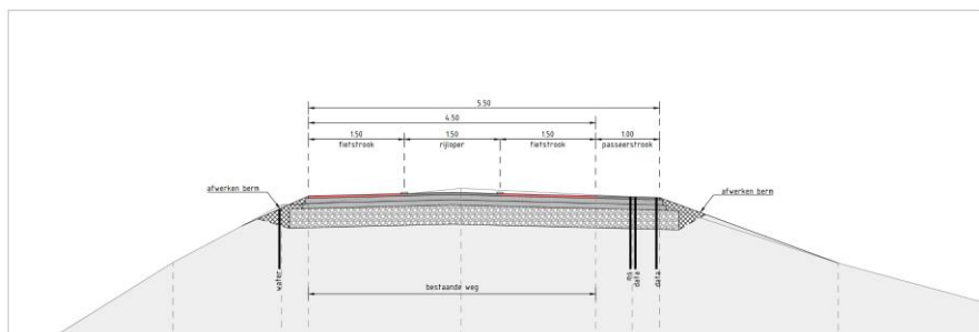
Principeprofiel Spaarndammerdijk schaal 1:50
