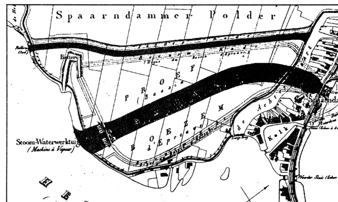
Detail van kaart II "Het Stoomgemaal te Spaarndam 10 oktober 1843" (Uit: Gevers van Endegeest).
